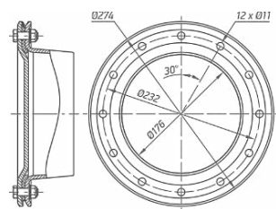
Flange DN180
